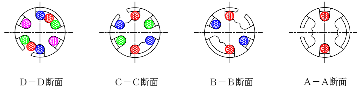
断面図 S=1/2
